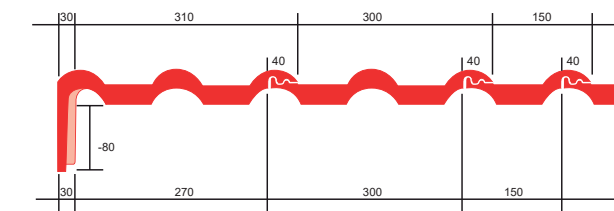
Krycí šířka levé krajové tašky u štítu = 31,0 cm
