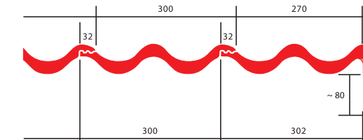
Krycí šířka pravé krajové tašky u štítu = 27,0 cm
