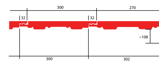
Krycí šířka pravé krajové tašky u štítu = 27,0 cm (12 cm poloviční taška)
