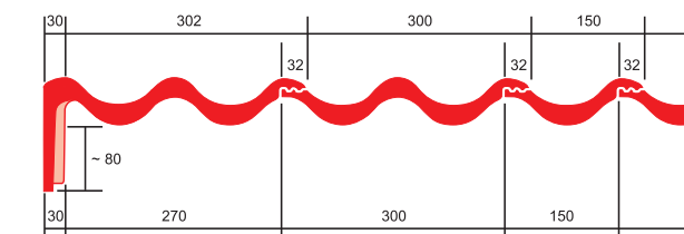
Krycí šířka levé krajové tašky u štítu = 30,2 cm
