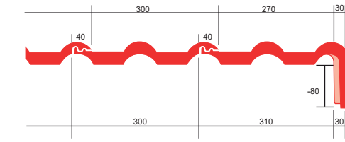
Krycí šířka pravé krajové tašky u štítu = 27,0 cm
