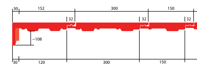
Krycí šířka levé krajové tašky u štítu = 30,2 cm (15,2 cm poloviční taška)
