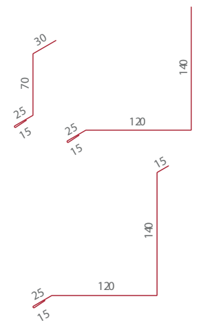
Lemování ke zdi F06
