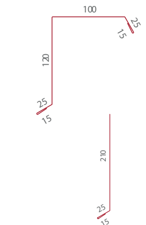
Závětrná lišta boční F02
