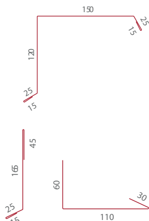
Závětrná lišta široká F03
