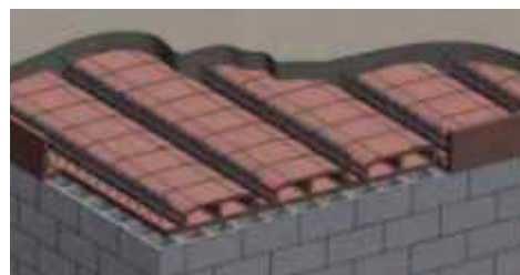
Řez stropem - věncová tvarovka KB STROP XC
