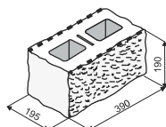
KB 7-21 B GRIND
