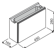
Lidovka hladká průběžná
