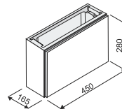
Lidovka hladká koncová
