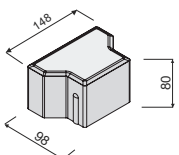
UNIKOST PŮLKA 80 mm
