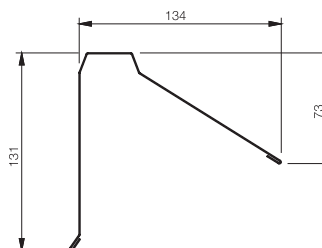
OVKSRP Přechodový plech – vikýře, dl. 2000 mm
