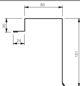
VISRP25 Štítové lemování, dl. 2000 mm
