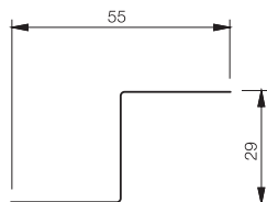
C2SRP Kotevní profil – napojení, dl. 2000 mm
