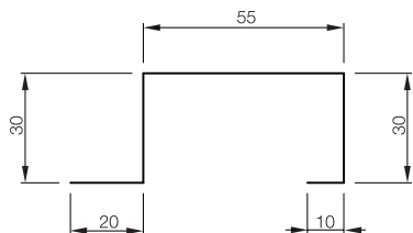
C1SRP25 Kotvící přípravek, dl. 485 mm
