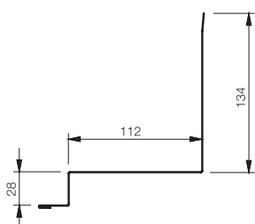
VISK - závětrná lišta pro taškovou krytinu, dl. 2000 mm
