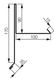
VISK-GL - závětrná lišta pro krytinu Goodlock, dl. 2000 mm
