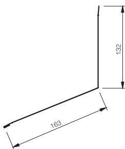
VISRP25 Štítové lemování, dl. 2000 mm
