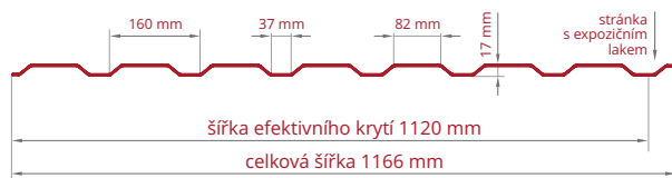
Fasádní profil
