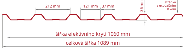
Střešní profil
