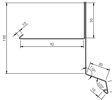
okapnice pod fólii
