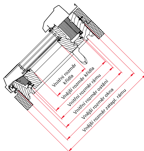
Řez B-B
