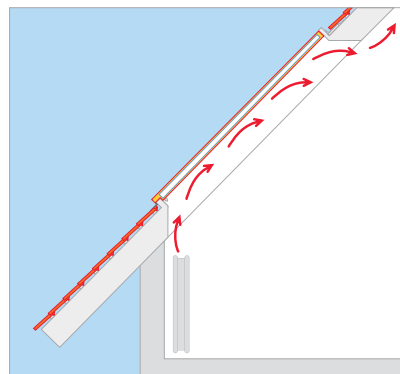
Proudění vzduchu podél okna při správné montáži vnitřního ostění
