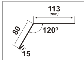
Guttatop Klasik okapové lemování
