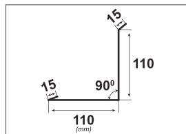
Guttatop Klasik lemování ke zdi spodní
