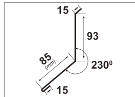
Guttatop Klasik lemování ke zdi vrchní
