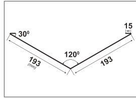
Guttatop Klasik úžlabí
