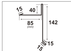
Guttatop Klasik štitové lemování spodní
