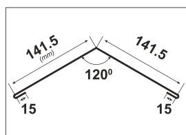
Guttatop Klasik hřebenáč hranatý
