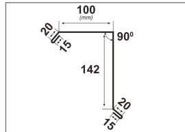
Guttatop Klasik štitové lemování vrchní
