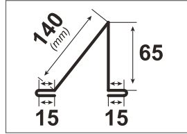
Guttatop Klasik sněhová zábrana
