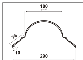
Guttatop Klasik hřebenáč oblý
