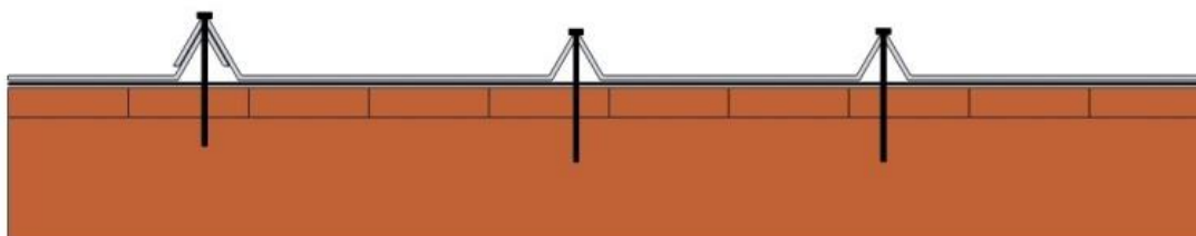
Kotvení hliníkovým hřebíkem s EPDM podložkou do horní vlny
