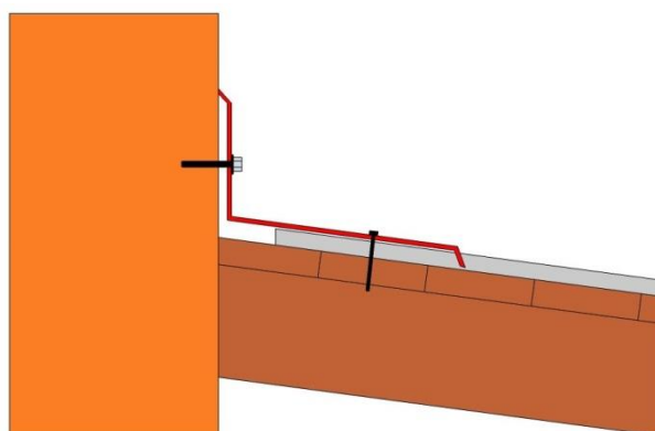
Výkres 7: Lišta ke zdi čelní - horní
