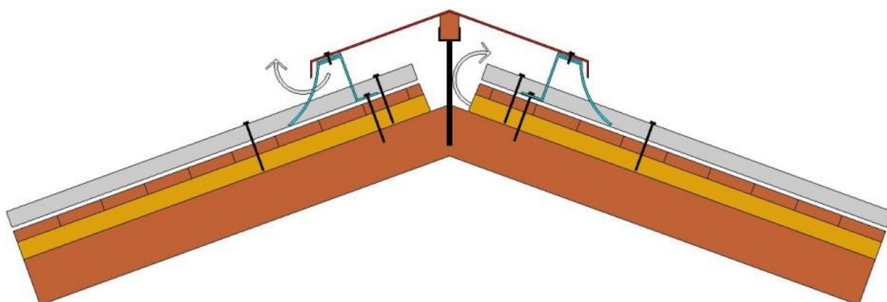
Výkres 2b: Detail větraného hřebenáče
