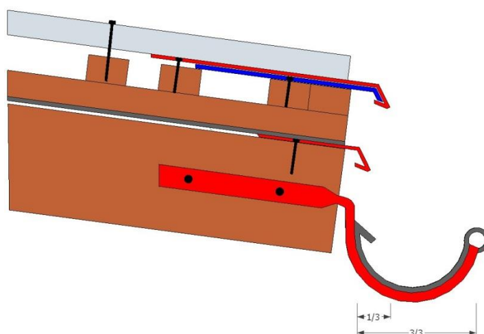
Výkres 1b: Detail odkapní hrany u větrané střešní skladby
