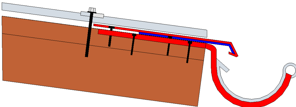
Výkres 1: Detail okapní hrany
