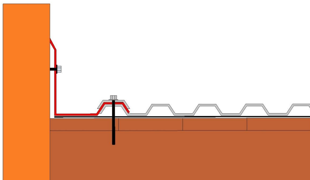
Výkres 6a: Boční lišta
