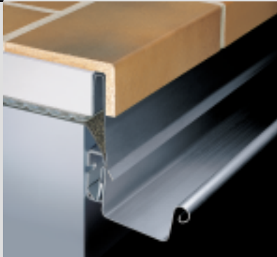
RHEINZINK®-balkonový zástrčný žlab
