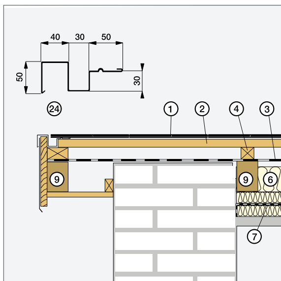
Plechové lemování okraje tříplášťové střešy s přesahem
