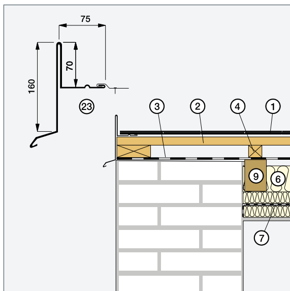
Plechové lemování okraje tříplášťové střešy bez přesahu
