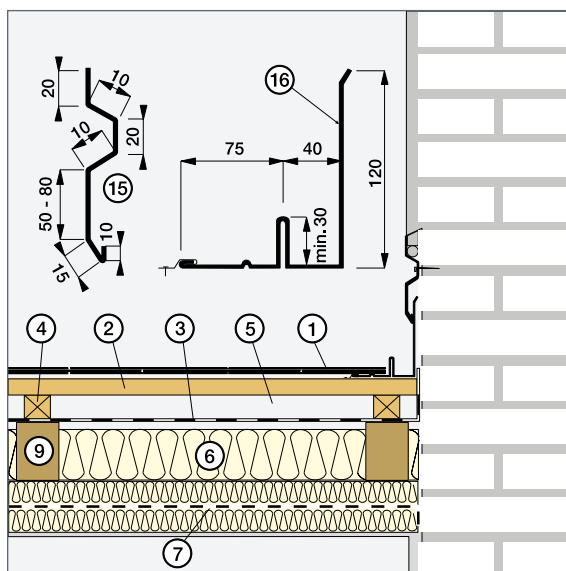
Plechové lemování okraje nadezdívky tříplášťové střešy
