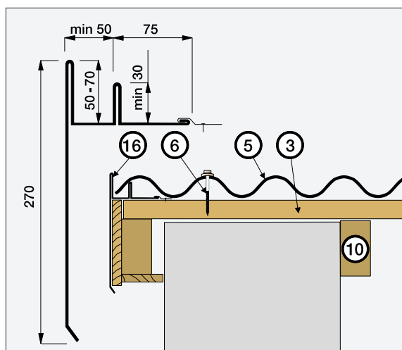
Plechové lemování okraje střešky
