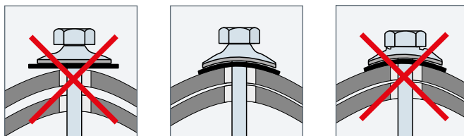
1. Správné dotažení upevňovacích šroubů
