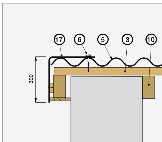
Lemování střešky úhelníkovým hřebenačem
