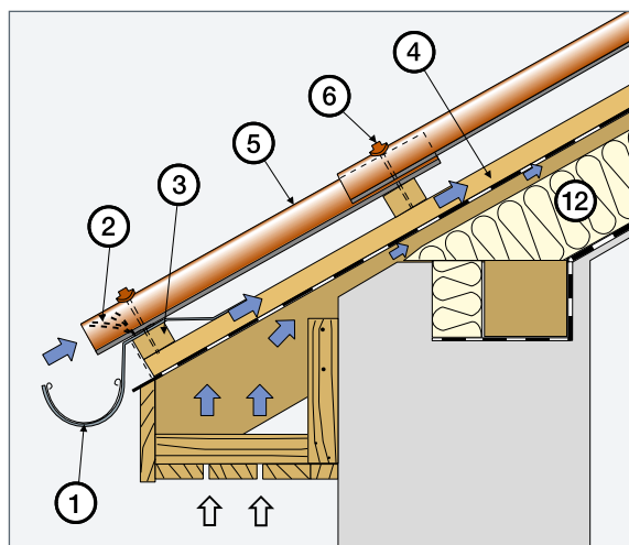
Okap střešky
