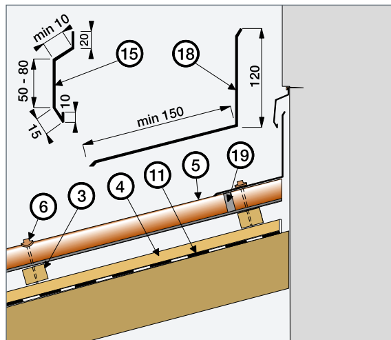
Plechový přechod střešky ke zdivu
