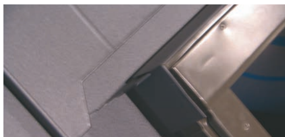
Osazení zadní části oplechování z hladkého plechu a uchycení třetí šablony zaháknutím o toto oplechování.
