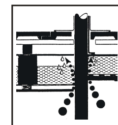
13 d/ Průnik stavebních konstrukcí střešním pláštěm: parotěsné a vzduchotěsné vrstvy nejsou dostatečně těsně napojeny na pronikající konstrukce
