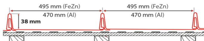
Schéma profilu:
