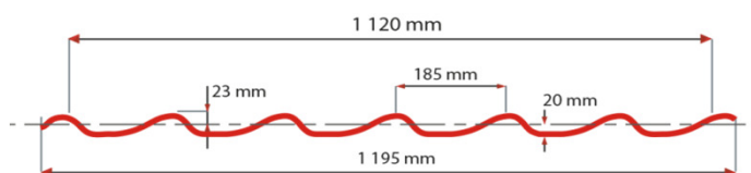
Schéma profilu:
