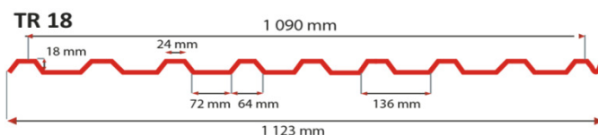
Schéma profilu:
