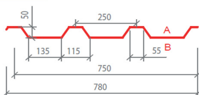
Rozvinutá šíře plechu - 1000 mm
