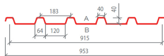
Rozvinutá šíře plechu - 1250 mm
