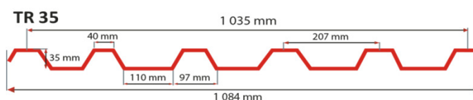
Schéma profilu:
